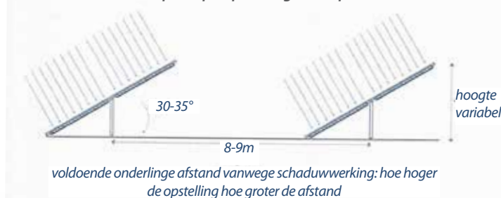
Voorbeeld van een principe opstelling zonnepanelen
