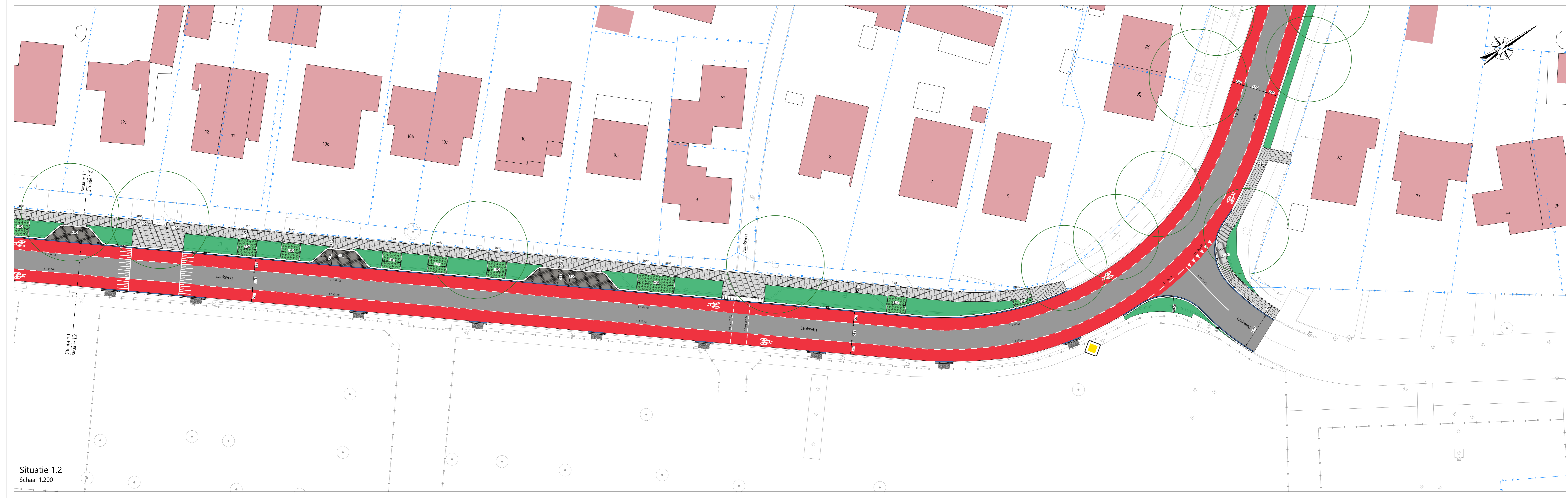
Situatie 1.1 Schaal 1:200
