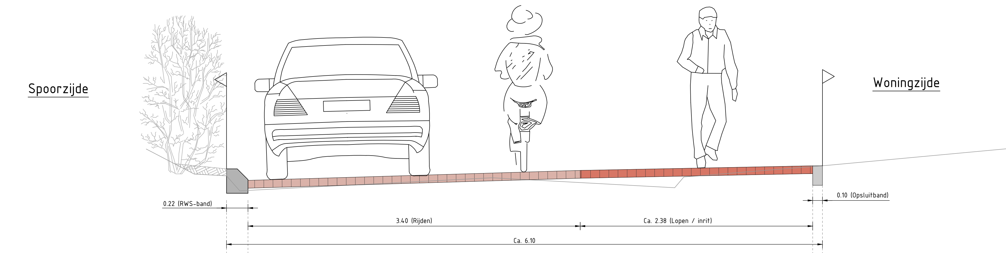
Principe dwarsprofiel B-B (t.p.v. inrit)
