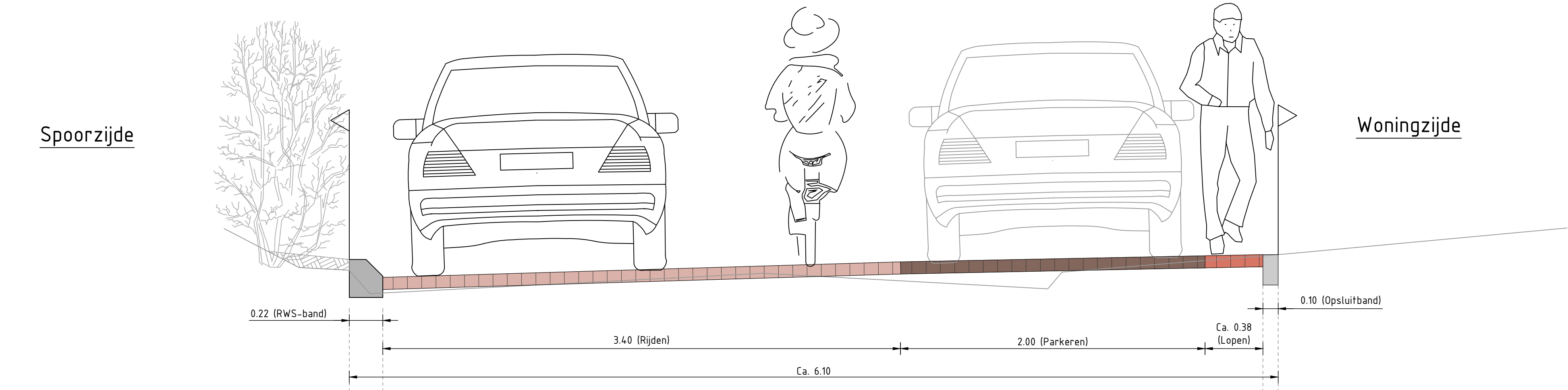
Principe dwarsprofiel A-A (t.p.v. parkeervak)
