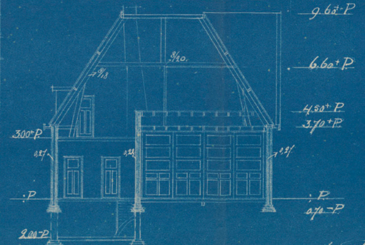
DWARSDOORSEDE
