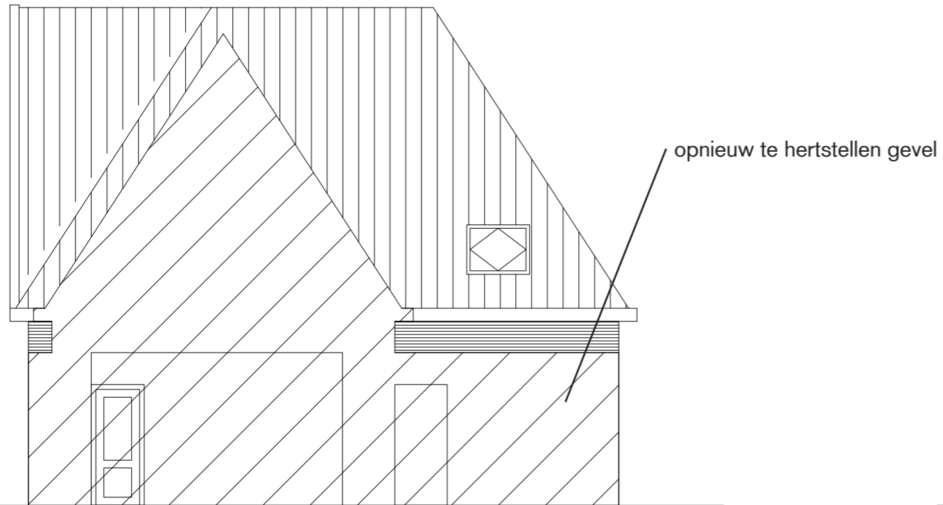
Zuidwest gevel
